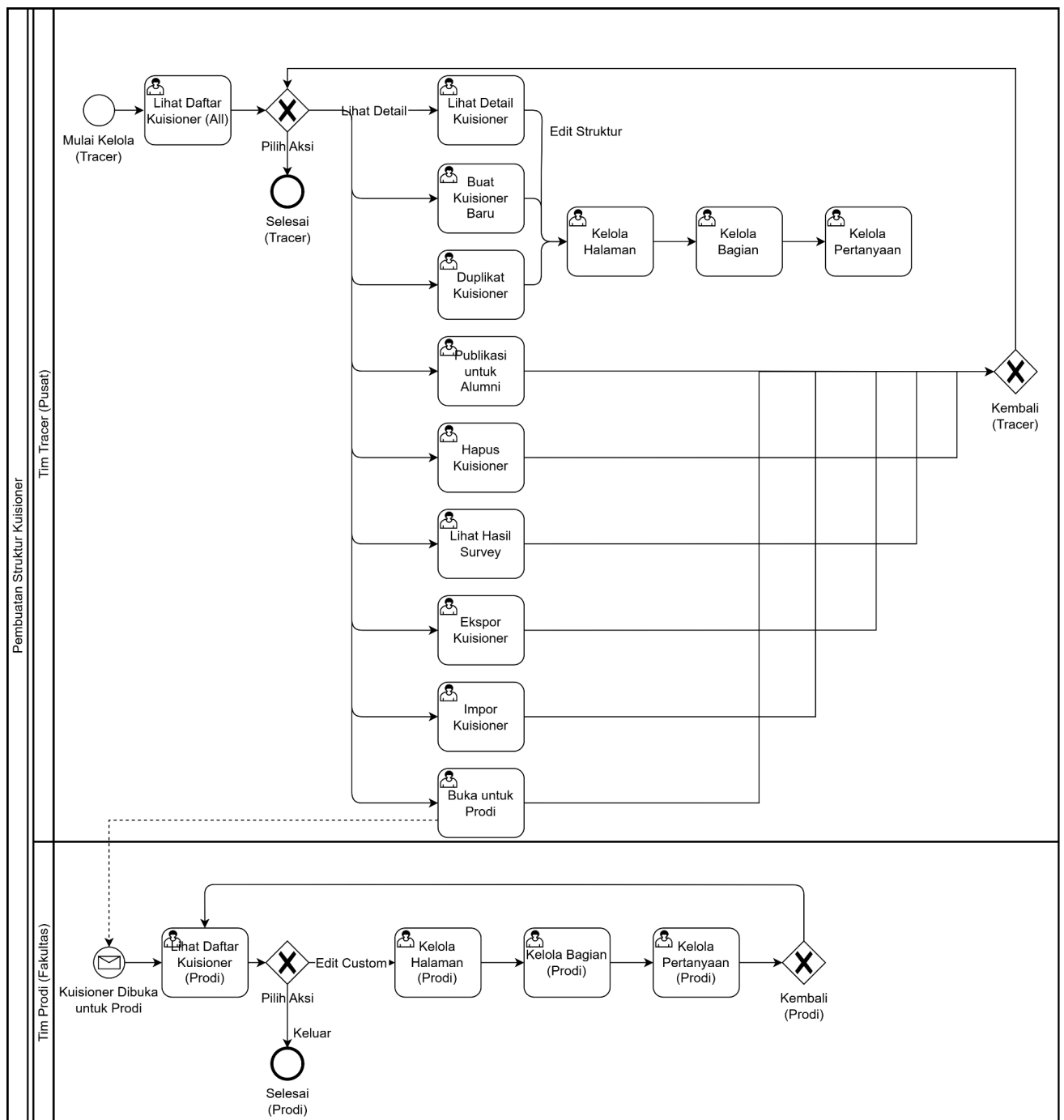
Gambar 3.7 Diagram Pembuatan Kuesioner
